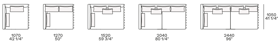
Terminale sx-dx
